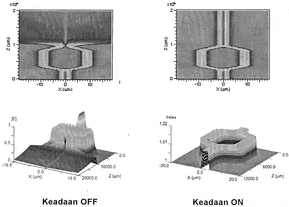
Rajah 2: Keadaan keluaran Pemodulat Keamatan Mach Zehnder
